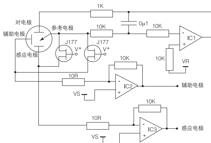
图10：四电极系列——标准操作电路图
